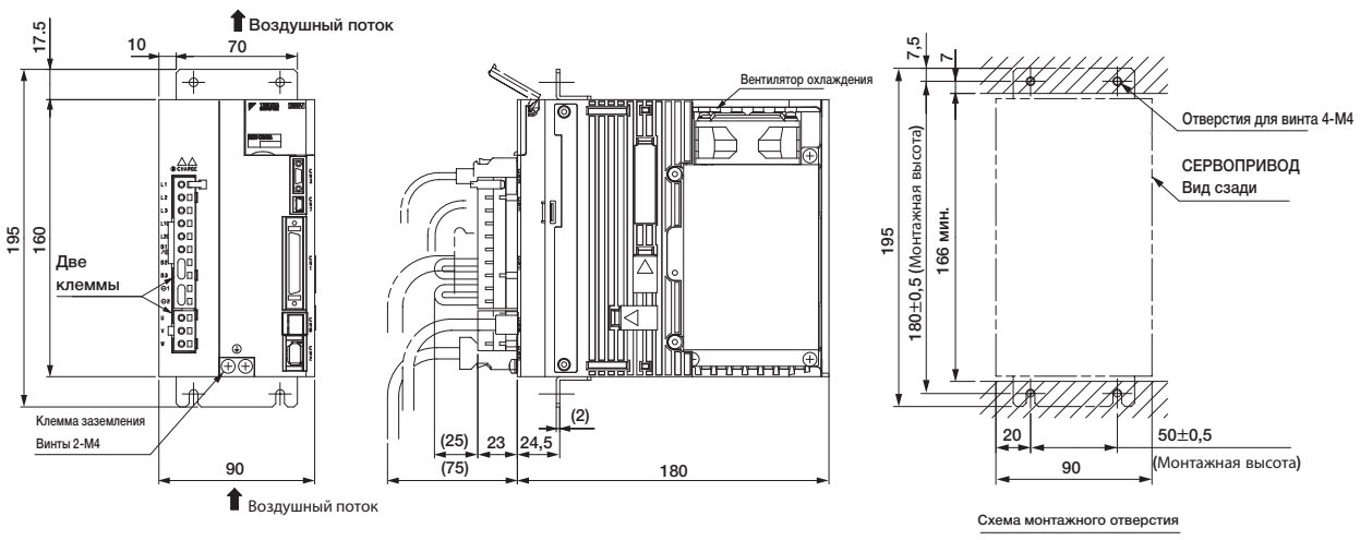
Приблиз. масса: 2,5 кг
