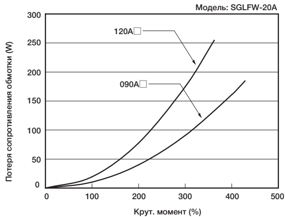
(h) Линейные сервод двигатели SGLFW
