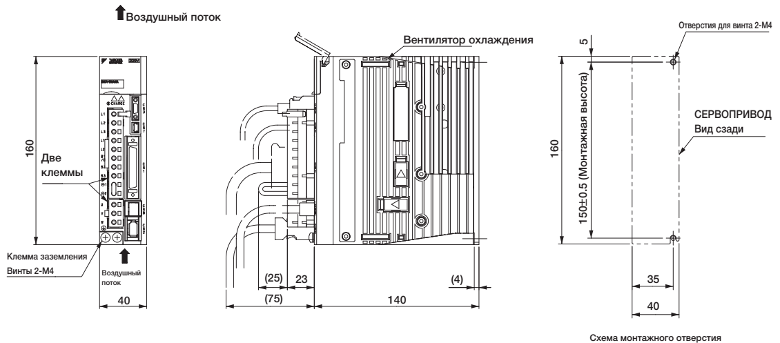
Схема монтажного отверстия
