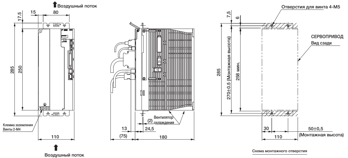
(12) Три фазы 400 В перем. напряжения, Модель: SGDВ-8R4D□□A001 и -120D□□A001
