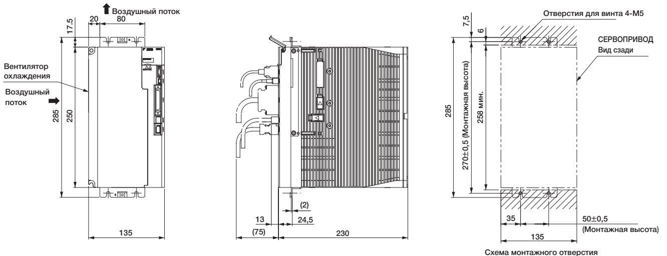
(13) Три фазы 400 В перем. напряжения, Модель: SGDВ-170D□□A001
