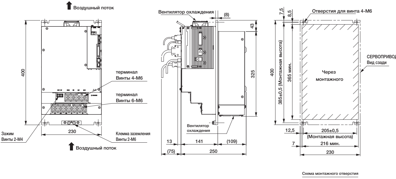
Приблиз. масса: 13,4 кг
