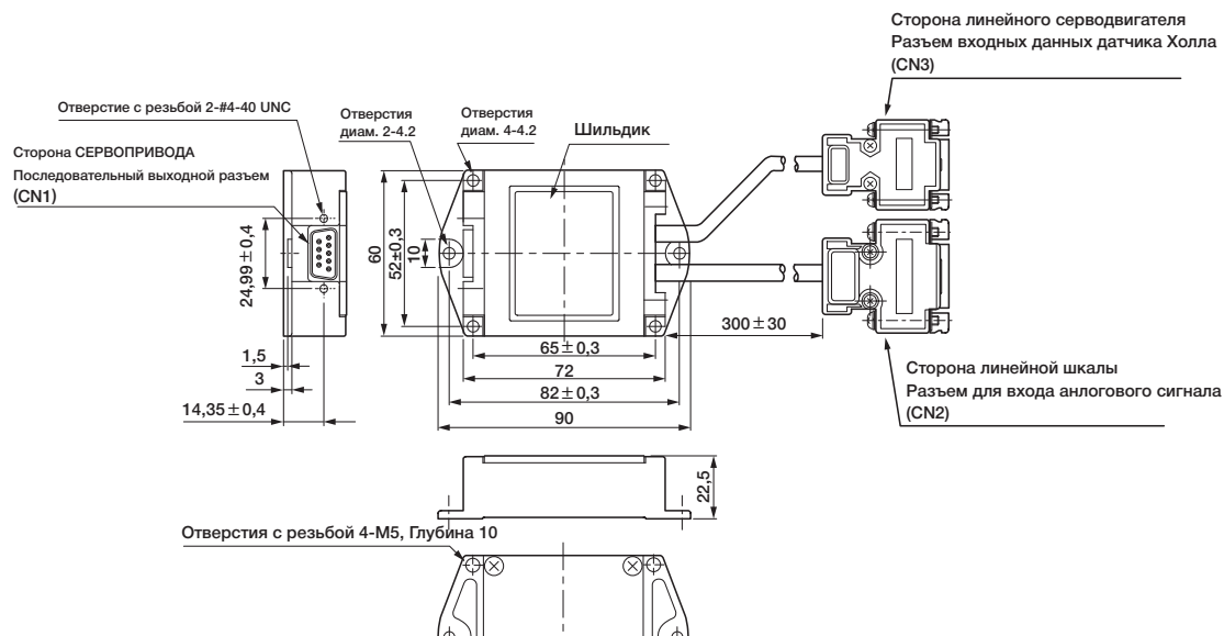
CN1 Сторона СЕРВОПРИВОДА Последовательный выходной разъем
