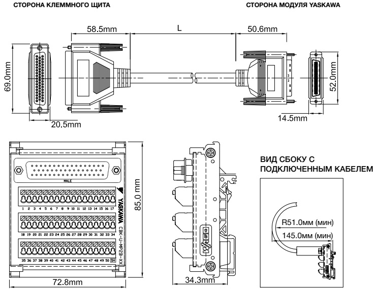
СВК-U-MP2B-XX Функциональная таблица для MP2600ies
