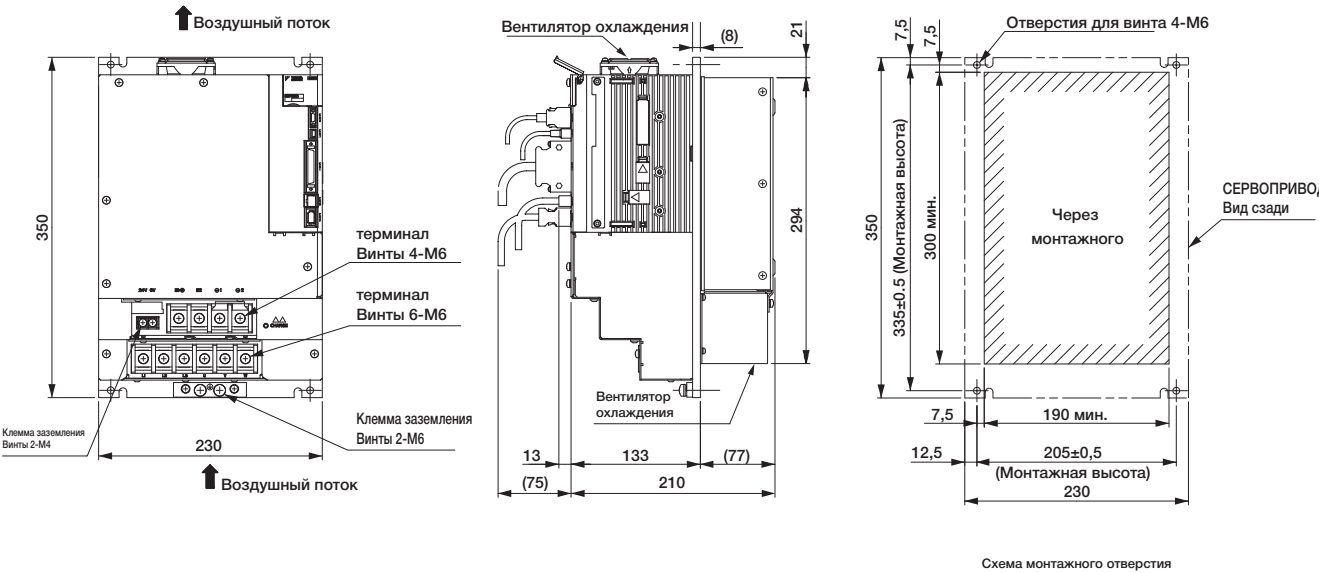
Приблиз. масса: 8,1 кг
