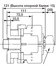
Для фронтального монтажа, контактная группа подключена.
