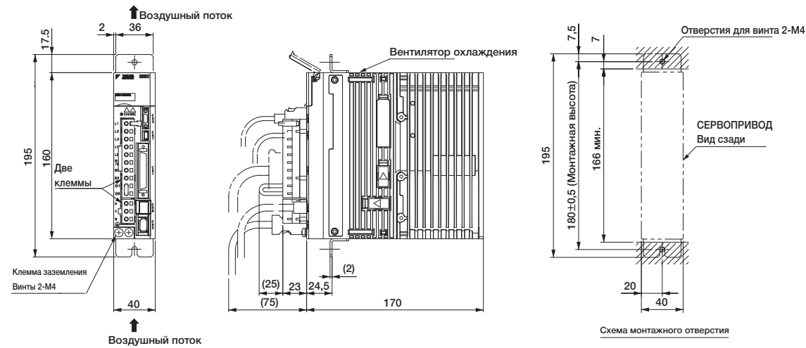
Приблиз. масса: 1,0 кг
