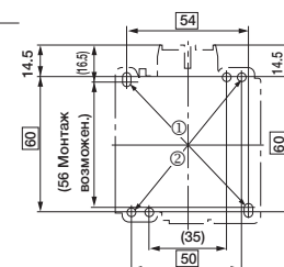
Размеры монтажных отверстий
