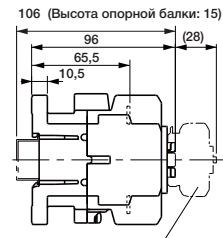
Для фронтального монтажа приобщены дополнит. контактные группы.
