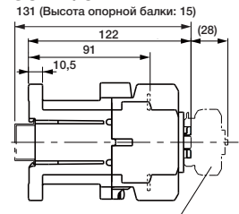
Для фронтального монтажа приобщены дополнит. контактные группы.
