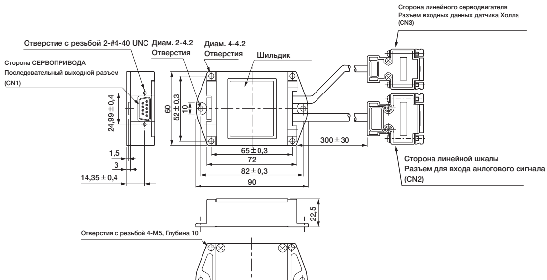
CN1 Сторона СЕРВОПРИВОДА Последовательный вывод данных
