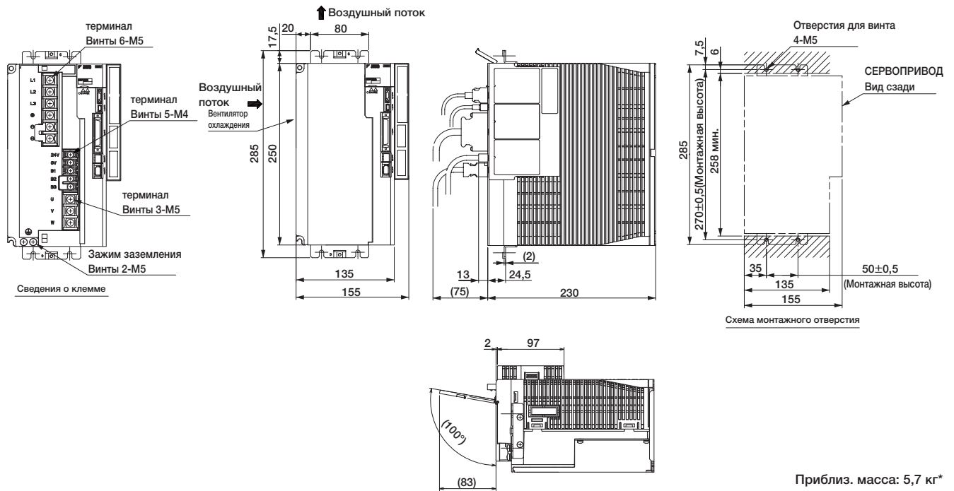
(14) Трехфазн. 400 В перем. напряжения, Модель: SGD V210D A001000 и SGD V260D A001000 (с вентиляционным трубопроводом)
