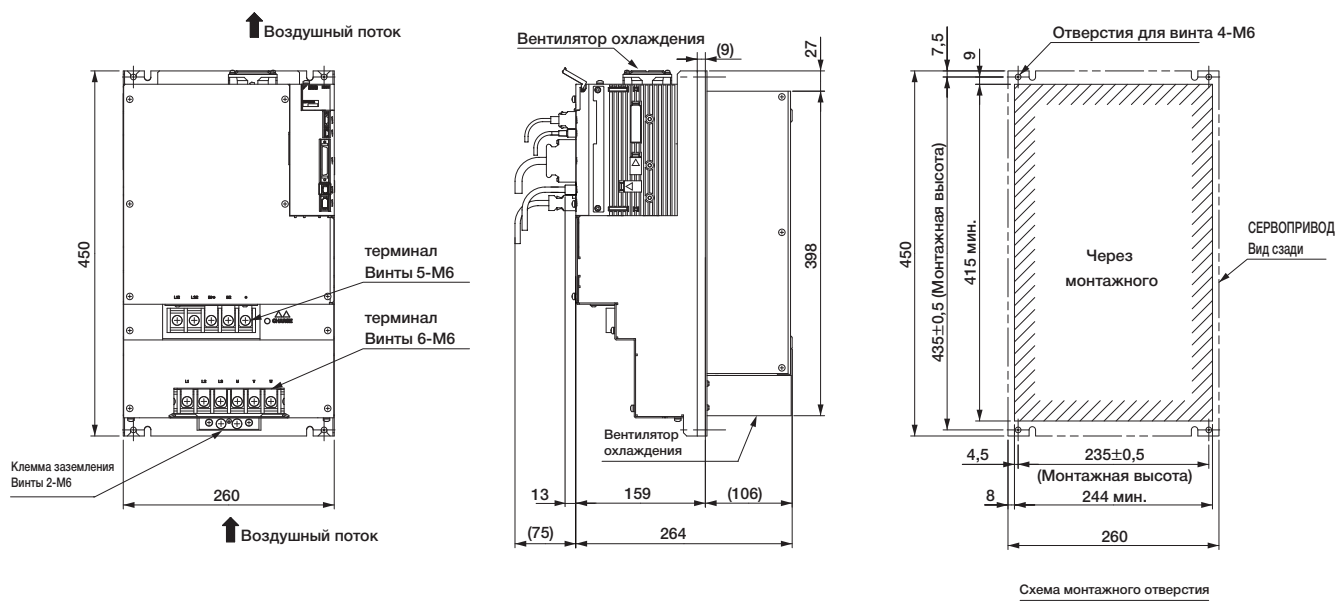
Приблиз. масса: 16,3 кг
