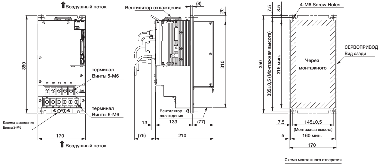
Приблиз. масса: 8,5 кг
