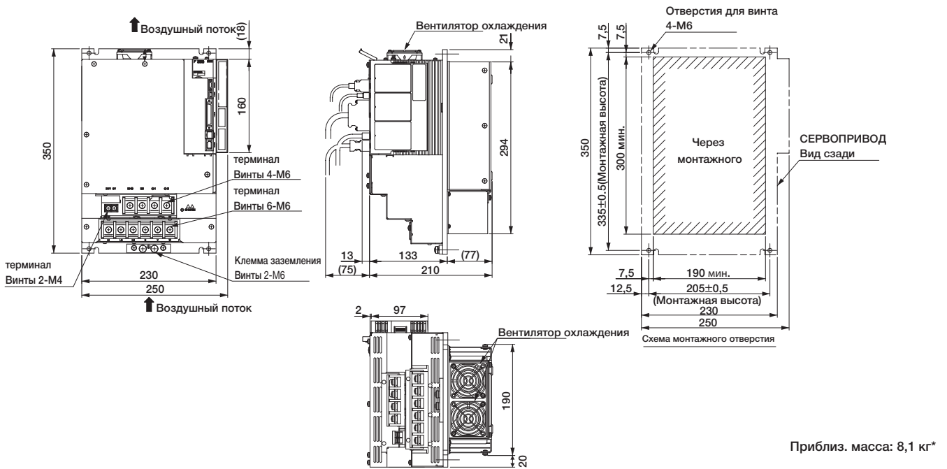
(14) Трехфазн. 400 В перем. напряжения, Модель: SGD V210D A001000 и SGD V260D A001000 (с вентиляционным трубопроводом)
