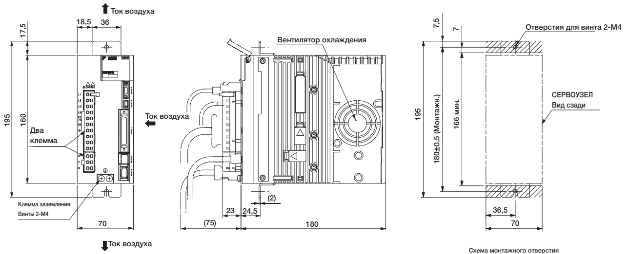
Схема монтажного отверстия
