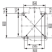
Размеры монтажных отверстий
