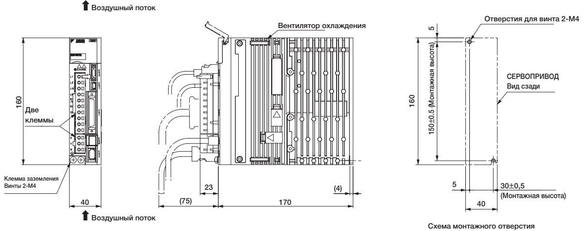
Схема монтажного отверстия
