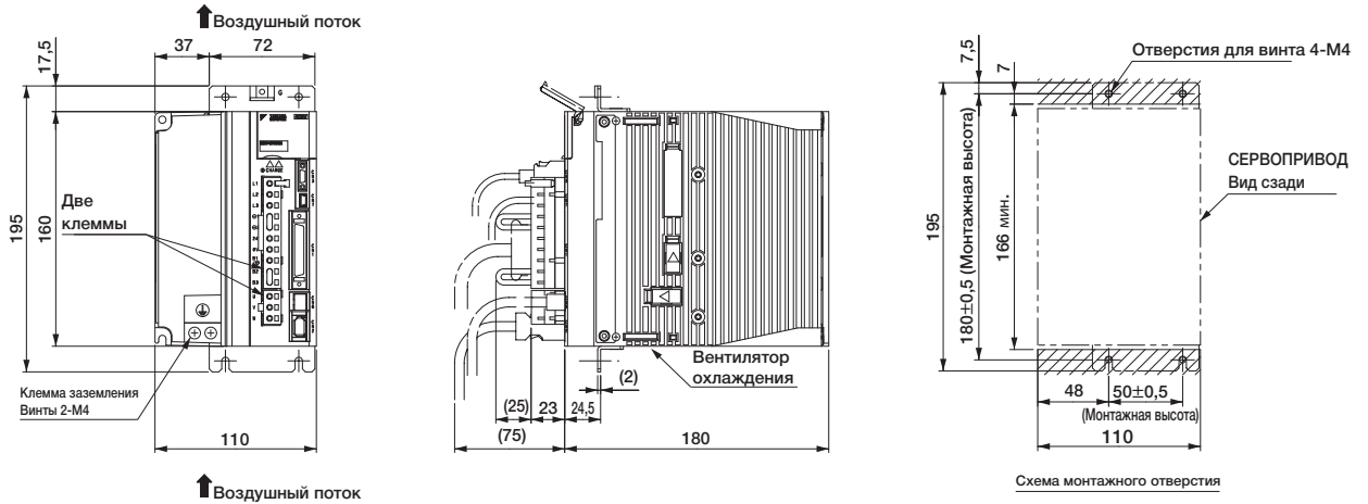
(11) Три фазы 400 В перем. напряжения, Модель: SGDВ-1R9D□□A001, -3R5D□□A001, и -5R4D□□A001
